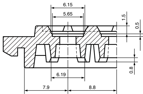
SEC. A-A
